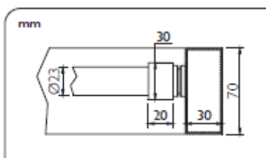
Fűtőtest méretei (mm)
